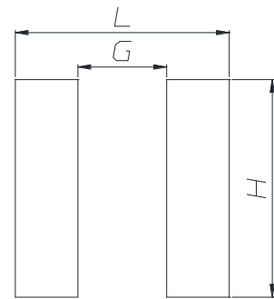
Land Pattern (Unit:mm)
