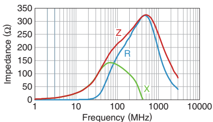
MPZ1608D101BTD25
